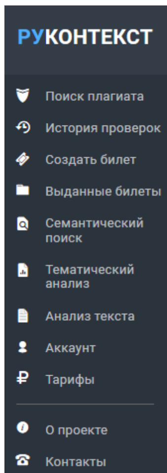
Рис.2.1.1. Главное меню
